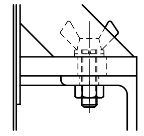
△蝶ボルト部詳細図 S = 1 : 2
