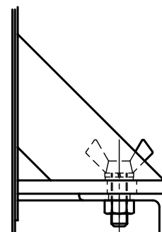
△蝶ボルト部詳細図 S = 1 : 4
