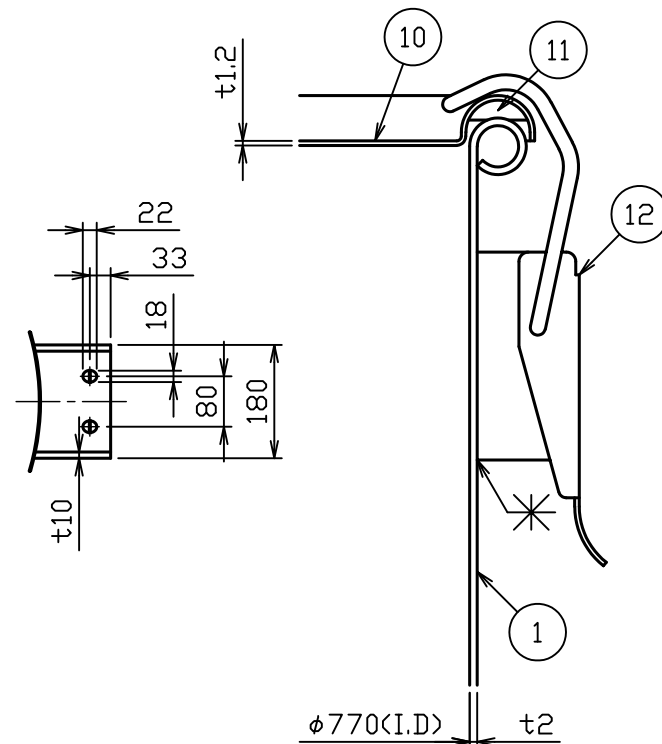
A部詳細図 S = 1 : 2
