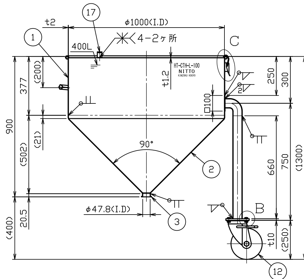
A-A断面図
