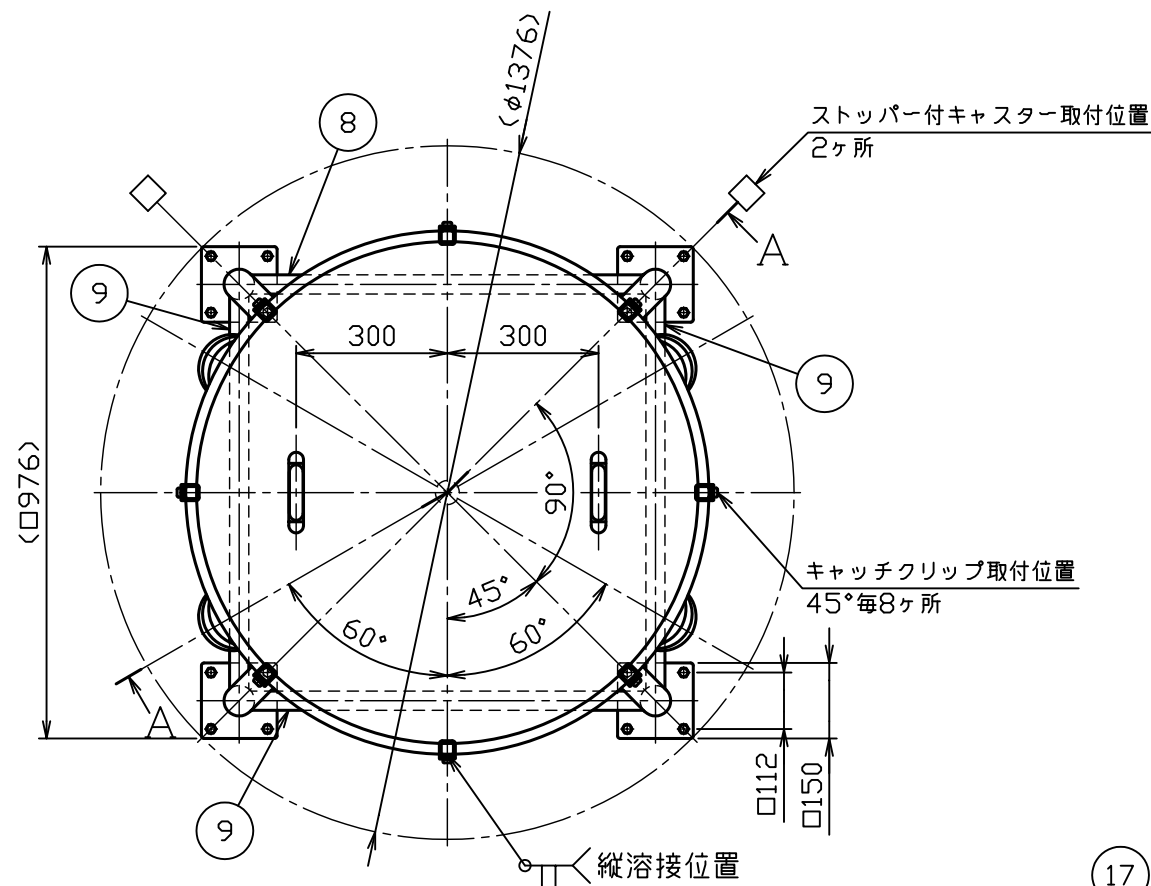
C部詳細図 S = 1 : 3
