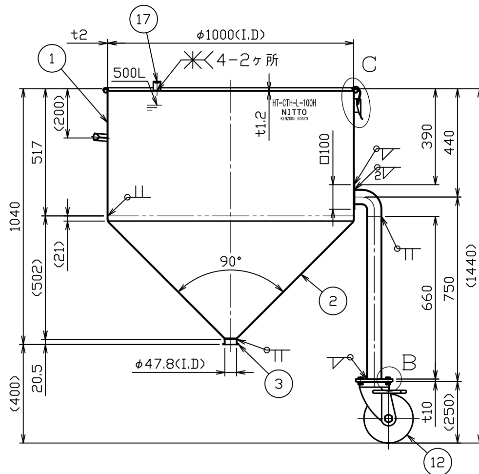
A-A断面図
