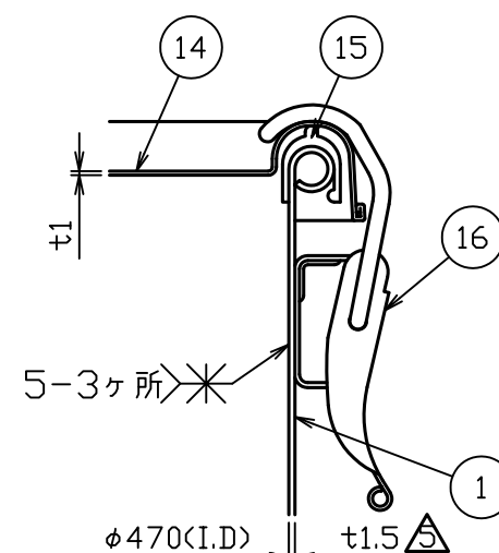
C-C断面図 S=1:2
