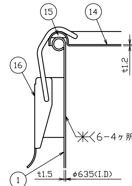
C部詳細図 S=1:2
