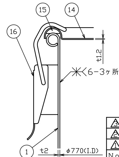
C部詳細図 S=1:2
