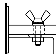
△ 蝶ボルト部詳細 S = 1 : 2
