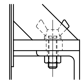
△蝶ボルト部詳細 S = 1 : 2
