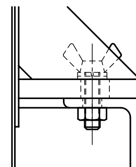
△蝶ボルト部詳細 S = 1 : 2
