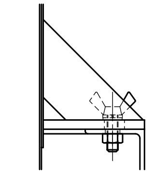
△蝶ボルト部詳細 S = 1 : 4
