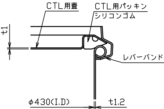
A部詳細図 S = 1 : 2
