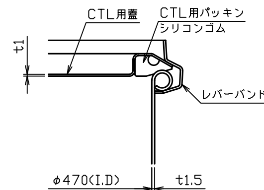
A部詳細図 S = 1 : 2
