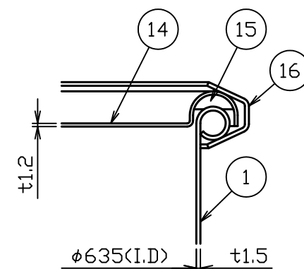
C部詳細図 S=1:2
