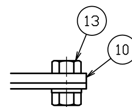
B部詳細図 S=1:2
