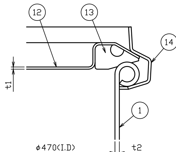
A部詳細図 S = 1 : 1
