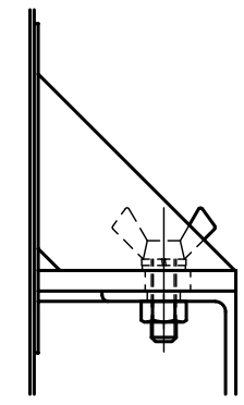
△蝶ボルト部詳細 S = 1 : 4
