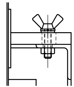
△蝶ボルト部詳細 S = 1 : 2
