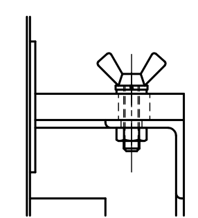
△蝶ボルト部詳細 S = 1 : 2
