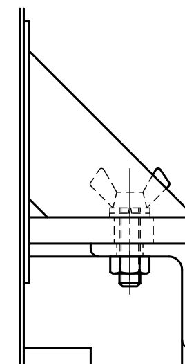
△蝶ボルト部詳細 S = 1 : 2
