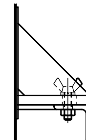
△ 蝶ボルト部詳細 S = 1 : 4
