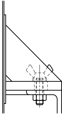
蝶ボルト部詳細図 S = 1 : 2
