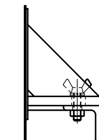
蝶ボルト部詳細図 S = 1 : 4
