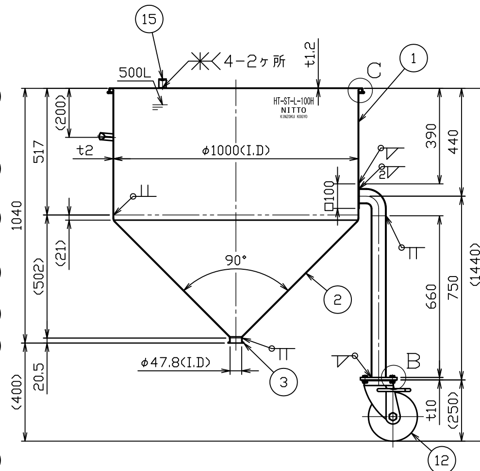
A-A断面図
