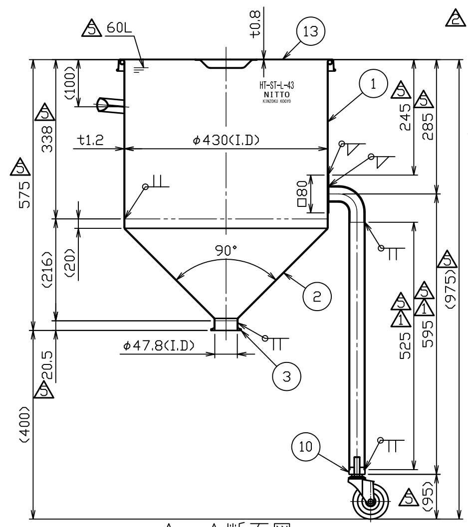
A-A断面図
