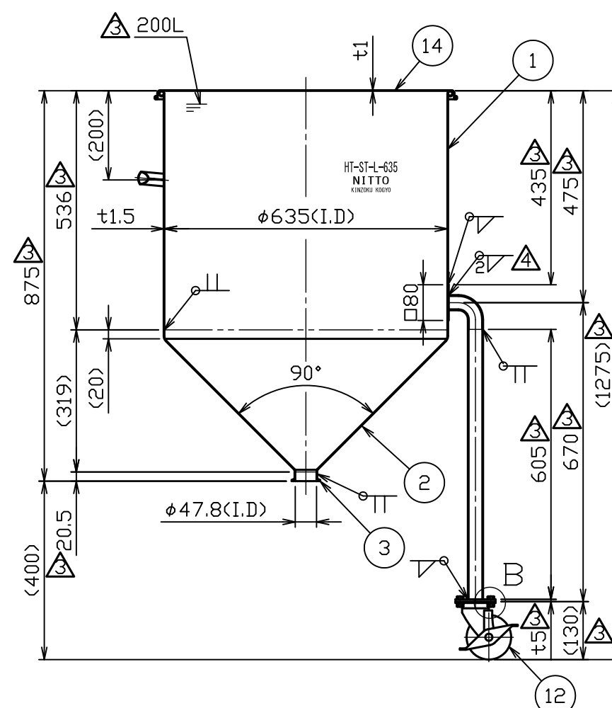
A-A断面図
