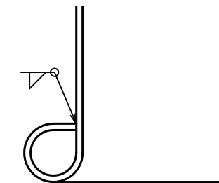
△ A部詳細図 S = 1 : 1
