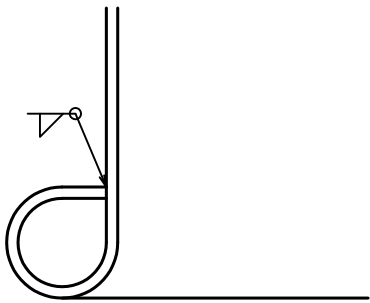
△ A部詳細図 S = 1 : 1
