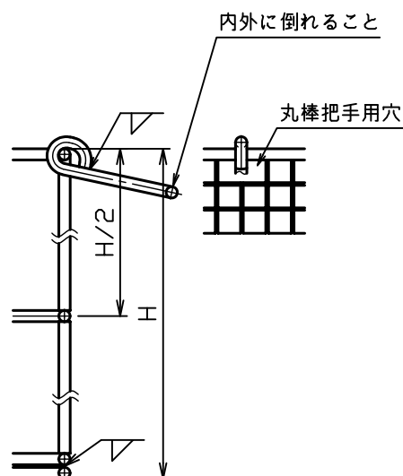
把手部詳細図 S = 1 : 3
