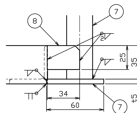
把手取付詳細図 S = 1 : 2
