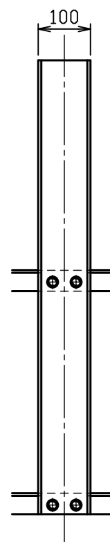
蝶ボルト部詳細図 S = 1 : 2
