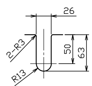
袴切り欠き詳細図
