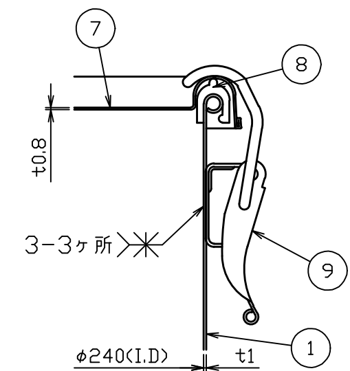
B部詳細図 S = 1 : 2
