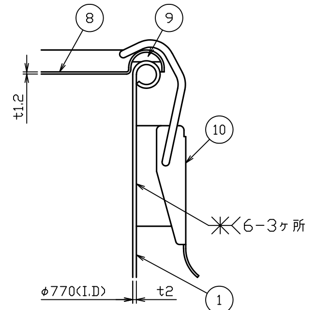
キャッチクリップ取付詳細図 S=1:2
