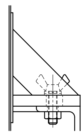
△ 蝶ボルト部詳細図 S = 1 : 2
