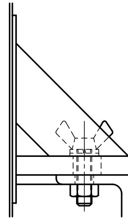
△ 蝶ボルト部詳細図 S = 1 : 2
