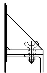
△ 蝶ボルト部詳細図 S = 1 : 4
