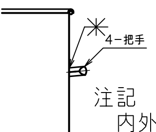
A部詳細図 S = 1 : 2
