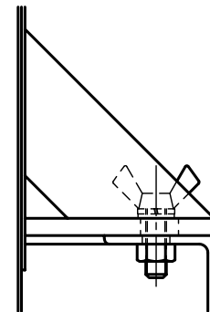
①蝶ボルト部詳細図 S = 1 : 4
