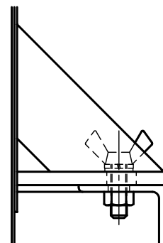
△蝶ボルト部詳細図 S = 1 : 4
