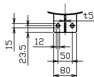
A部詳細図 S = 1 : 2
