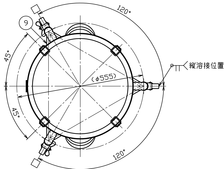
A部詳細図 S = 1 : 2
