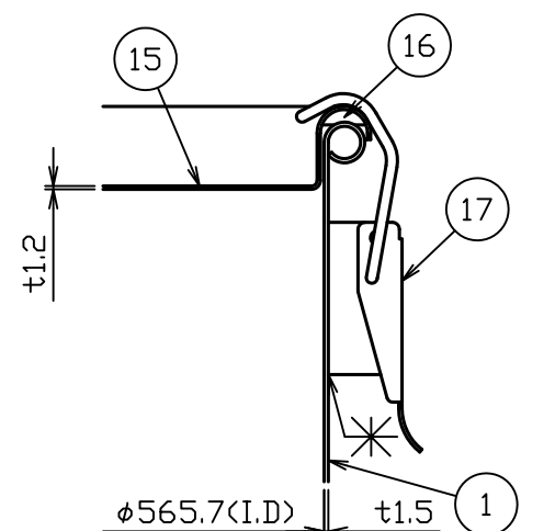
A部詳細図 S = 1 : 3
