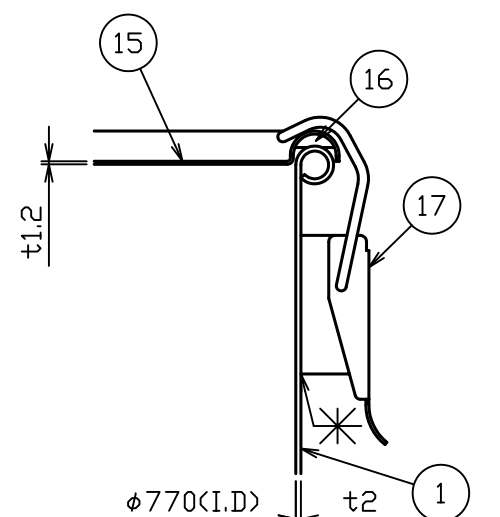
A部詳細図 S = 1 : 3
