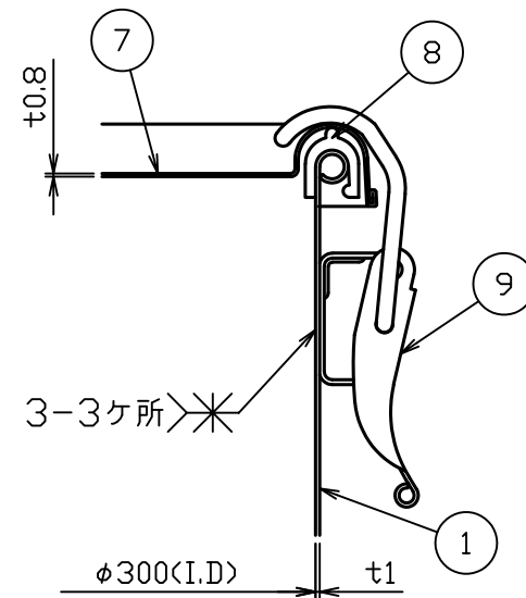
B-B断面图 S = 1 : 2
