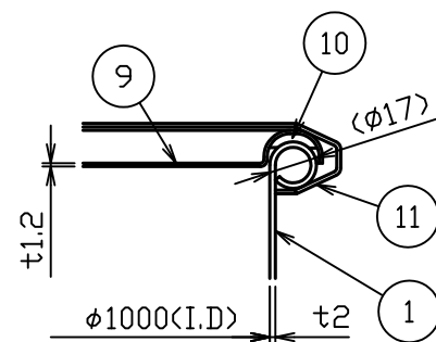
A部詳細図 S = 1 : 3
