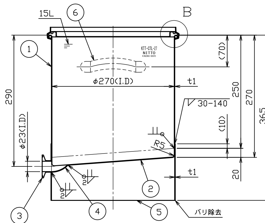
A-A断面図
