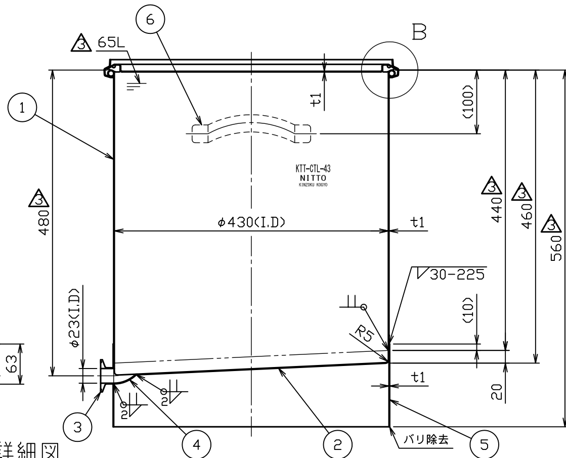
A-A断面図
