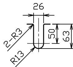
袴切り欠き詳細図
