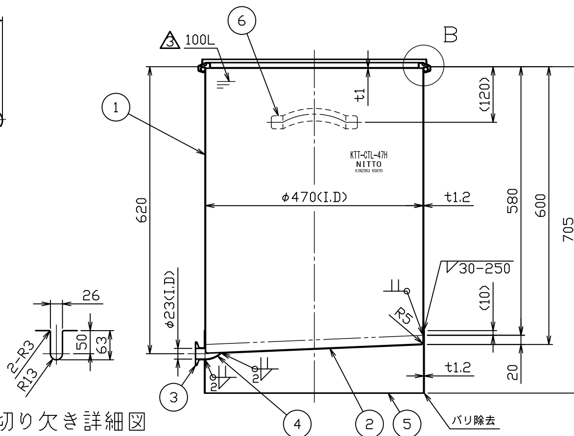
A-A断面图
