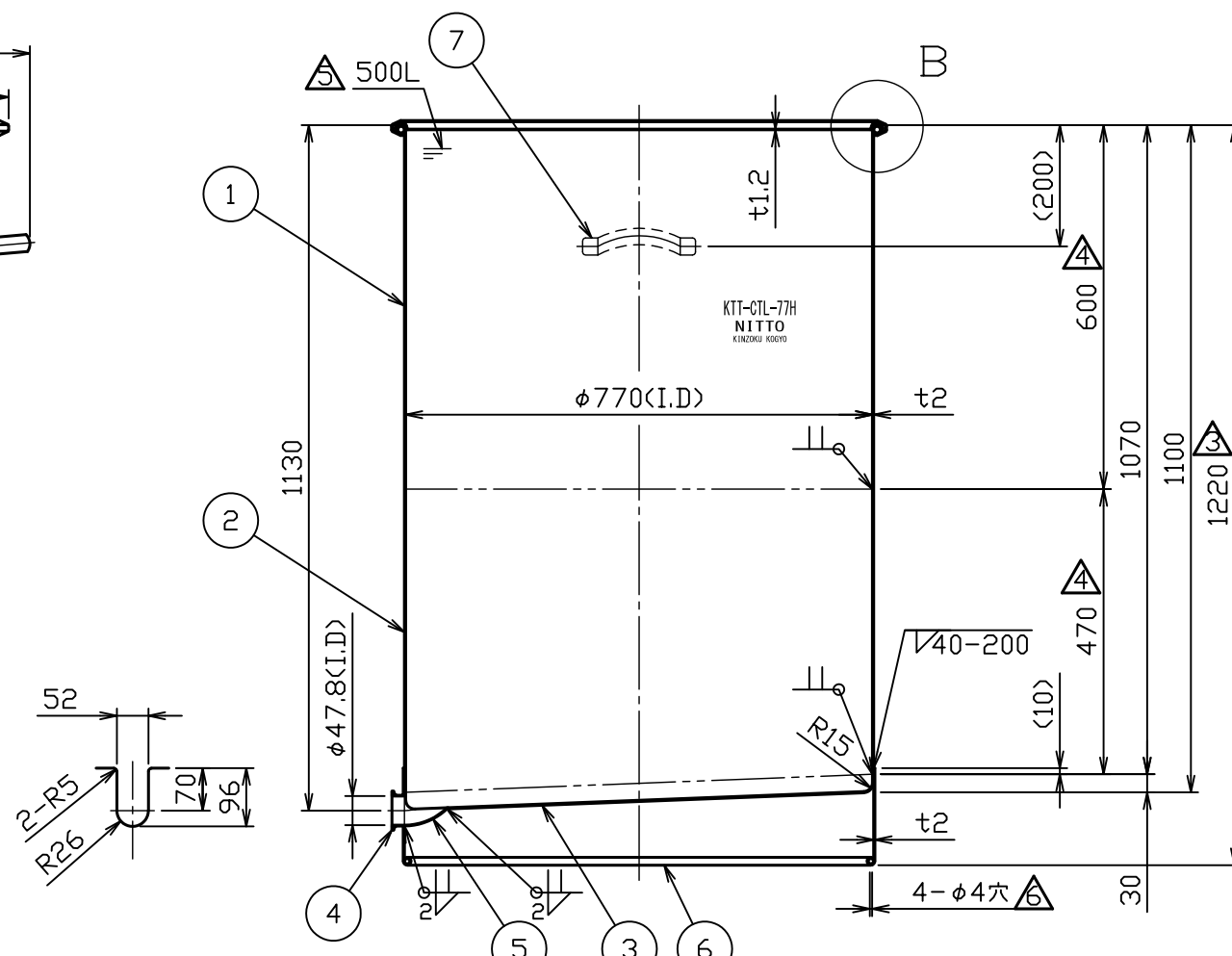
袴切り欠き詳細図
