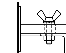
△ 蝶ボルト部詳細図 S = 1 : 2
