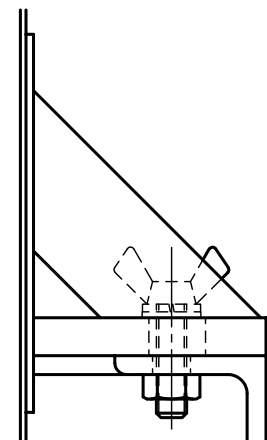
△ 蝶ボルト部詳細図 S = 1 : 2
